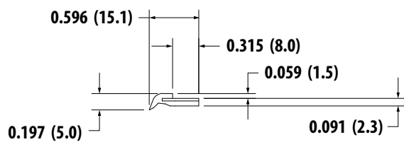
TFW-MA8/N6 (N6 Wiper)
